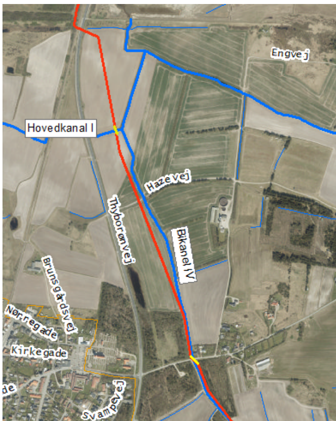
Figur 2: Kablet med markeret med rød linje og underboringerne med gul. Her krydses de offentlige vandløb Bikanal IV og Hovedkanal I
